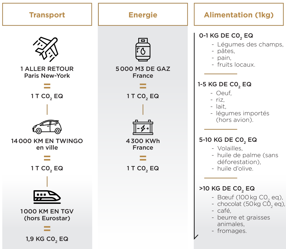
Figure 3. Exemple de l'impact carbone pour des activités du quotidien
