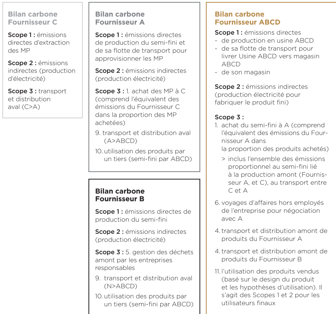
Figure 1. Bilan carbone pour une entreprise fictive ABCD (et ses fournisseurs)
